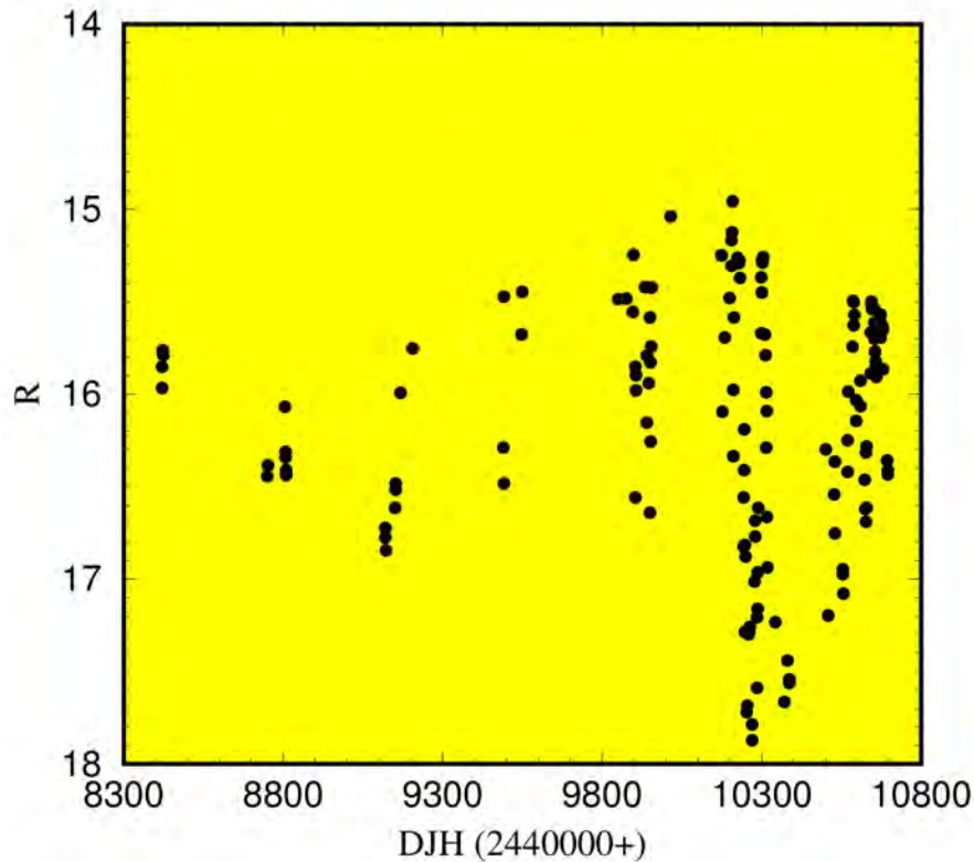
Figura 4.8 - Curva de luz de longa duração de V2116 Oph/GX1+4. Observações realizadas na banda R ao longo dos anos 1991-1997.
