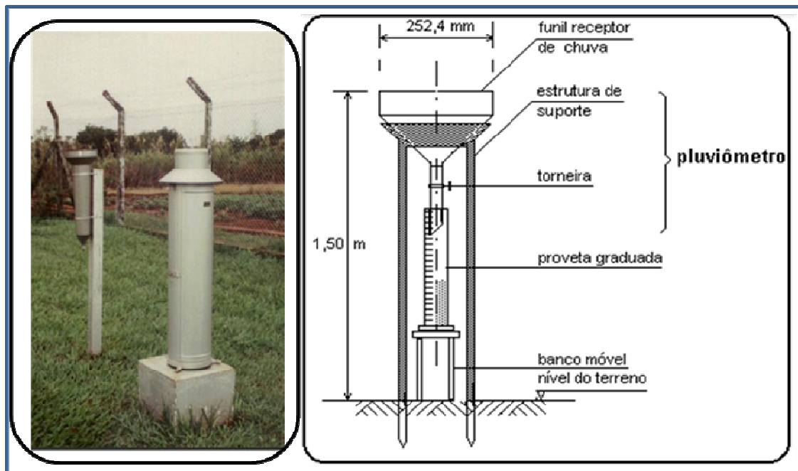
Fig. 7 – Pluviógrafo e pluviômetro e demonstração de como funciona o pluviômetro. Fonte: (adaptada) www.geocities.com/mpcarvalho_2000/pluviome.htm
