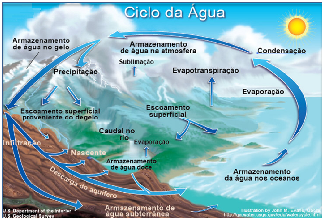
Fig. 5. – Ciclo da água
