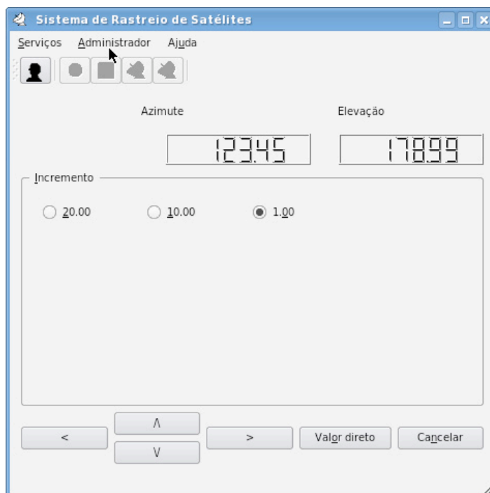
Figura 35: Tela para Movimentação manual da Antena
