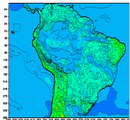
Cssf_aysS 17/12/06
