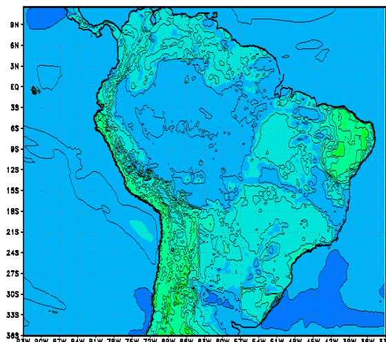
Cssf_oriS 17/12/06
