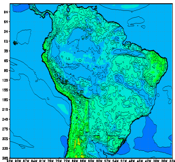
Cssf_aysF 17/12/06
