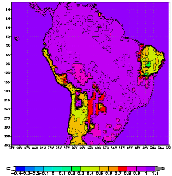
Smav_oriS 17/12/06
