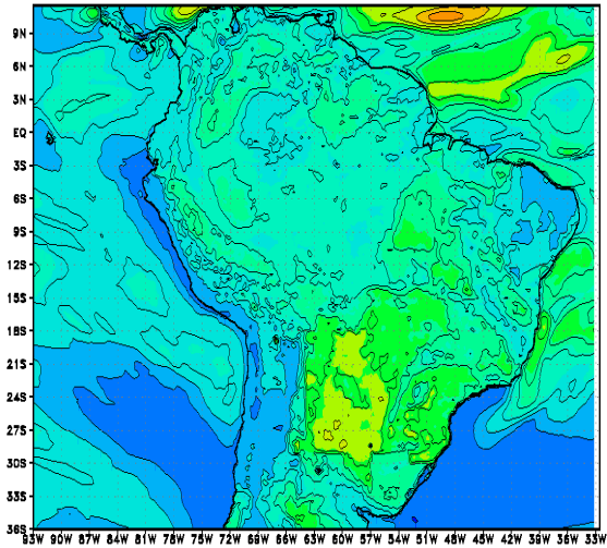
Clsf_oriS 17/12/06
