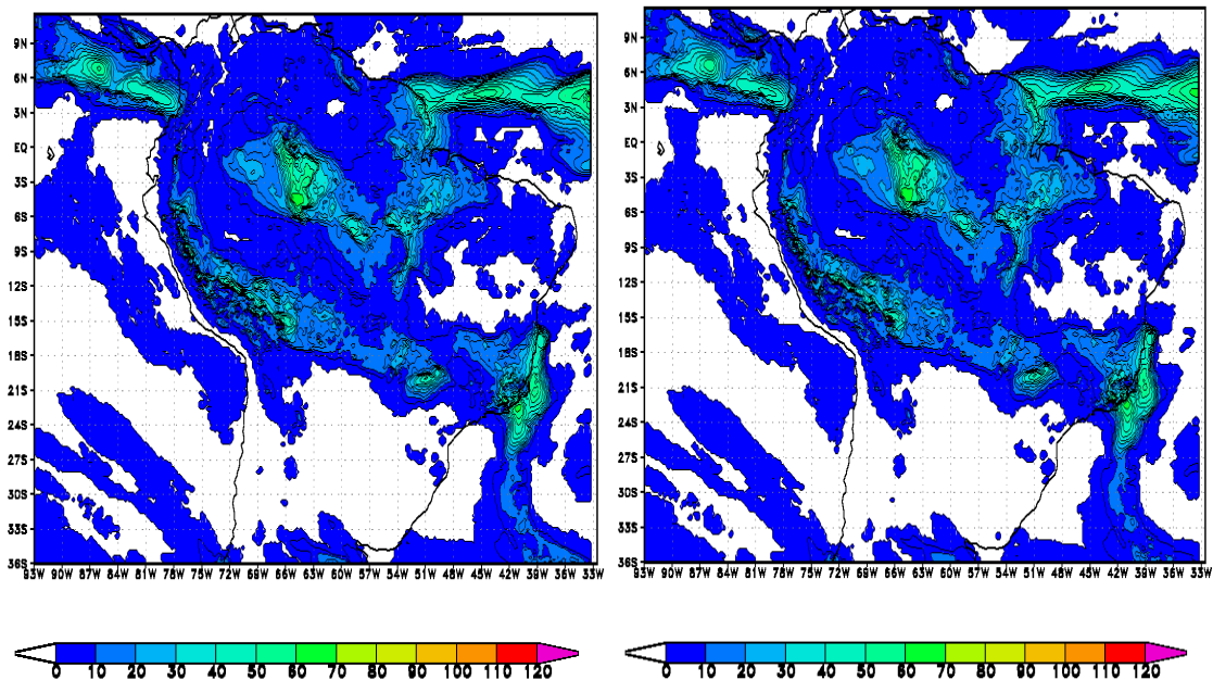
Prec_oriF 16/12/06
