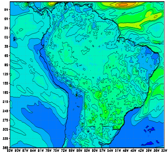
Clsf_aysS 17/12/06
