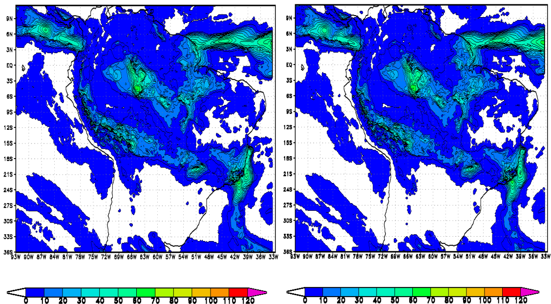
Figura 6: Precipitação acumulada nos dias 16 e 17. Imagens superiores correspondentes ao experimento CTRL, a da esquerda utilizando o modo previsão e a da direita em modo simulação. As imagens inferiores são idênticas as superiores, mas para o experimento AYS. Unidades: mm.
