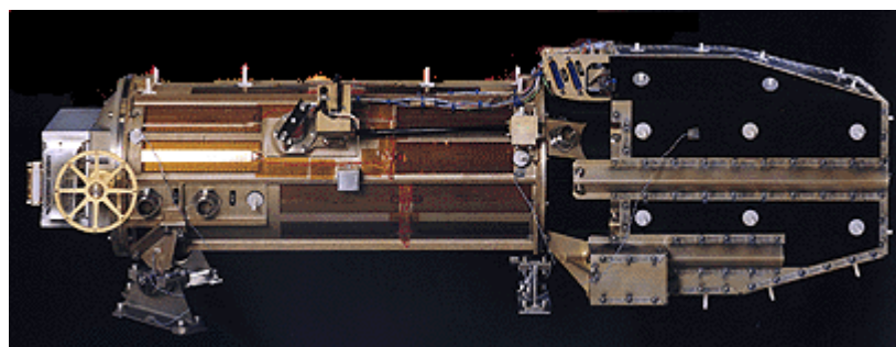
FIGURA 31: Imagem do telescópio EIT. FONTE: http://umbra.nascom.nasa.gov/eit
