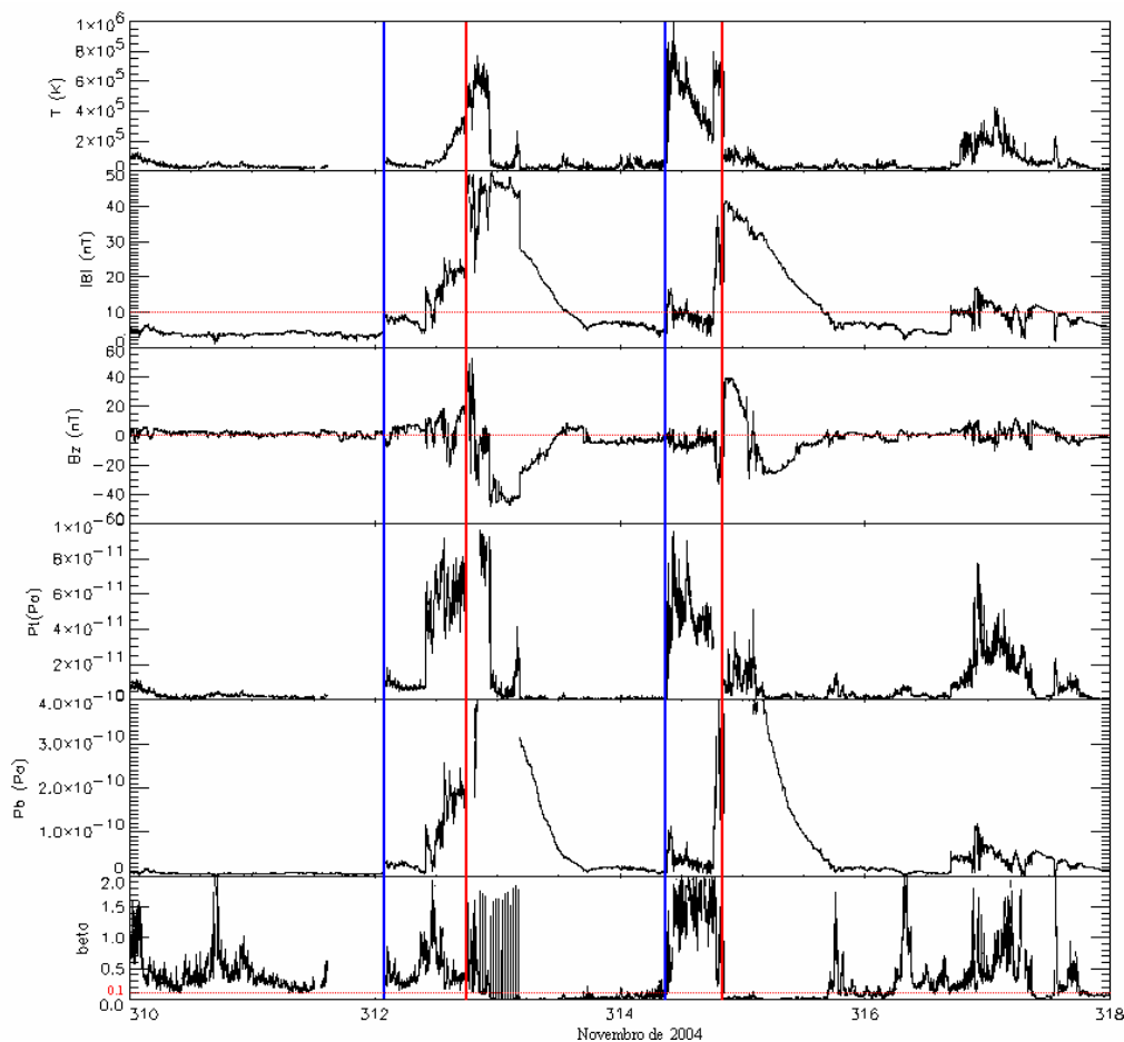
FIGURA 40: Painel de gráficos do meio interplanetário de novembro de 2004.
