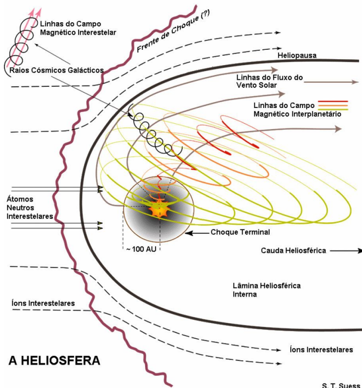
FIGURA 11: Esquema da heliosfera e suas principais características. FONTE: Modificado de http://canopy.lsmal.com/schryver/Public/homepage/coolstarimages4.html .
