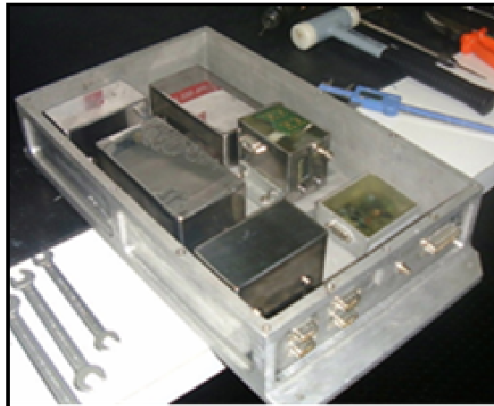
Figura 3: Estrutura na forma de caixa retangular Fonte: http://www.space.unopar.br/
