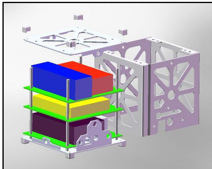
Figura 30: Vista explodida da arquitetura mecânica Fonte: Desenhado por Prochnow, S. L., 2008
