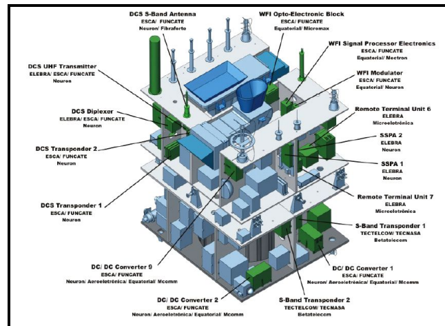
Figura 15: Arquitetura Mecânica do Satélite Cbers – 2 Fonte: www.inpe.br
