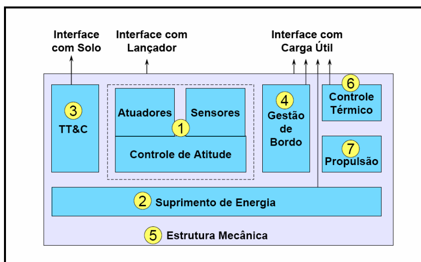
Figura 9: Diagrama de blocos dos subsistemas de um satélite
