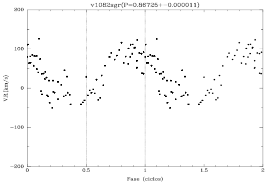
Figura 8: Diagrama de fase de V1082 Sgr para o período de (0.86725 \pm 0.00001) d.
