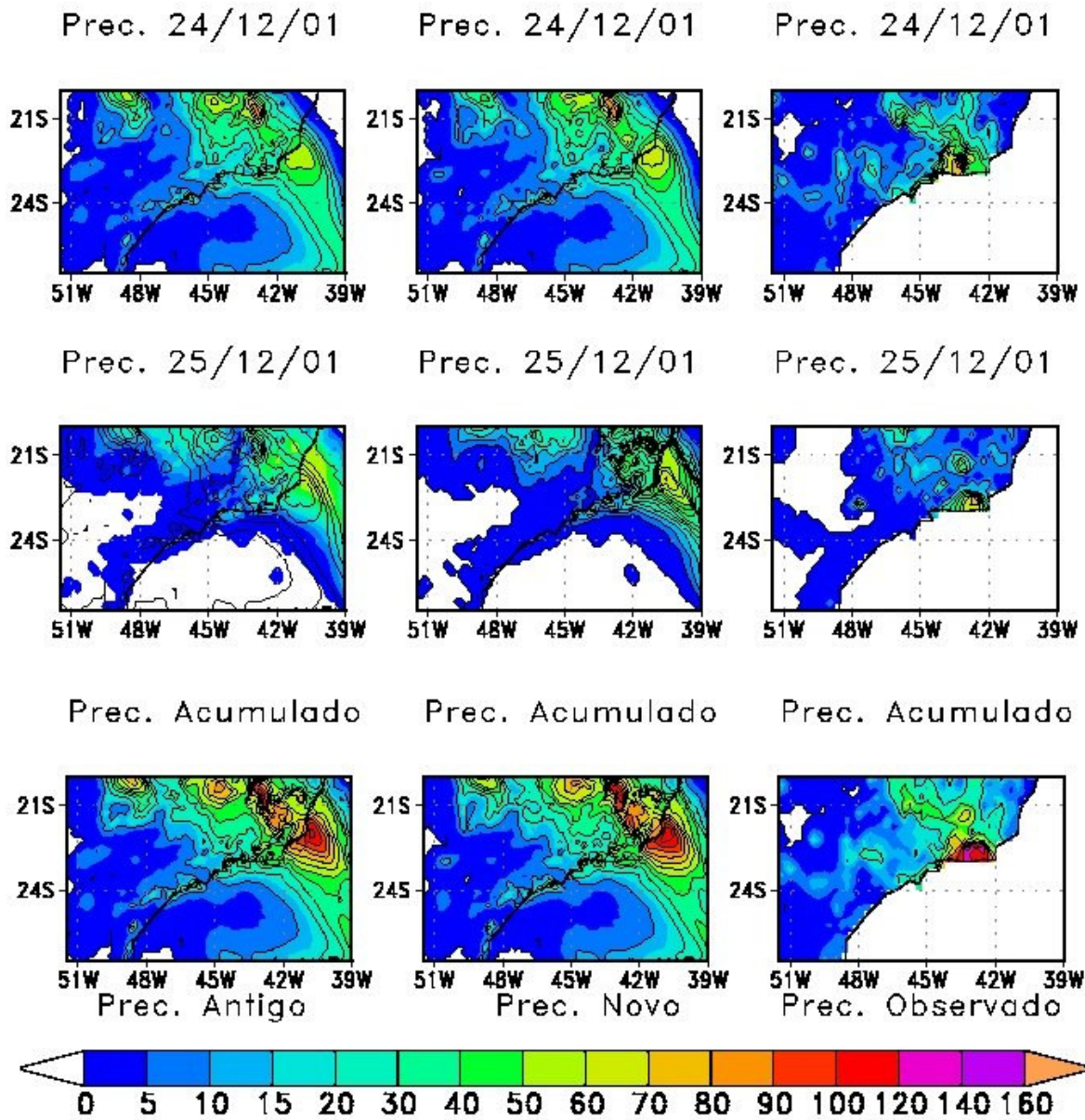
Figura 12 PRECIPITAÇÃO (mm)
