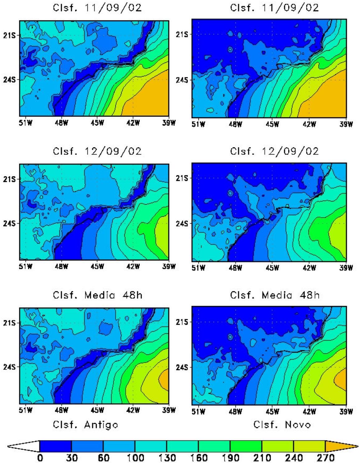
Figura 03: CALOR LATENTE(W/m2)
