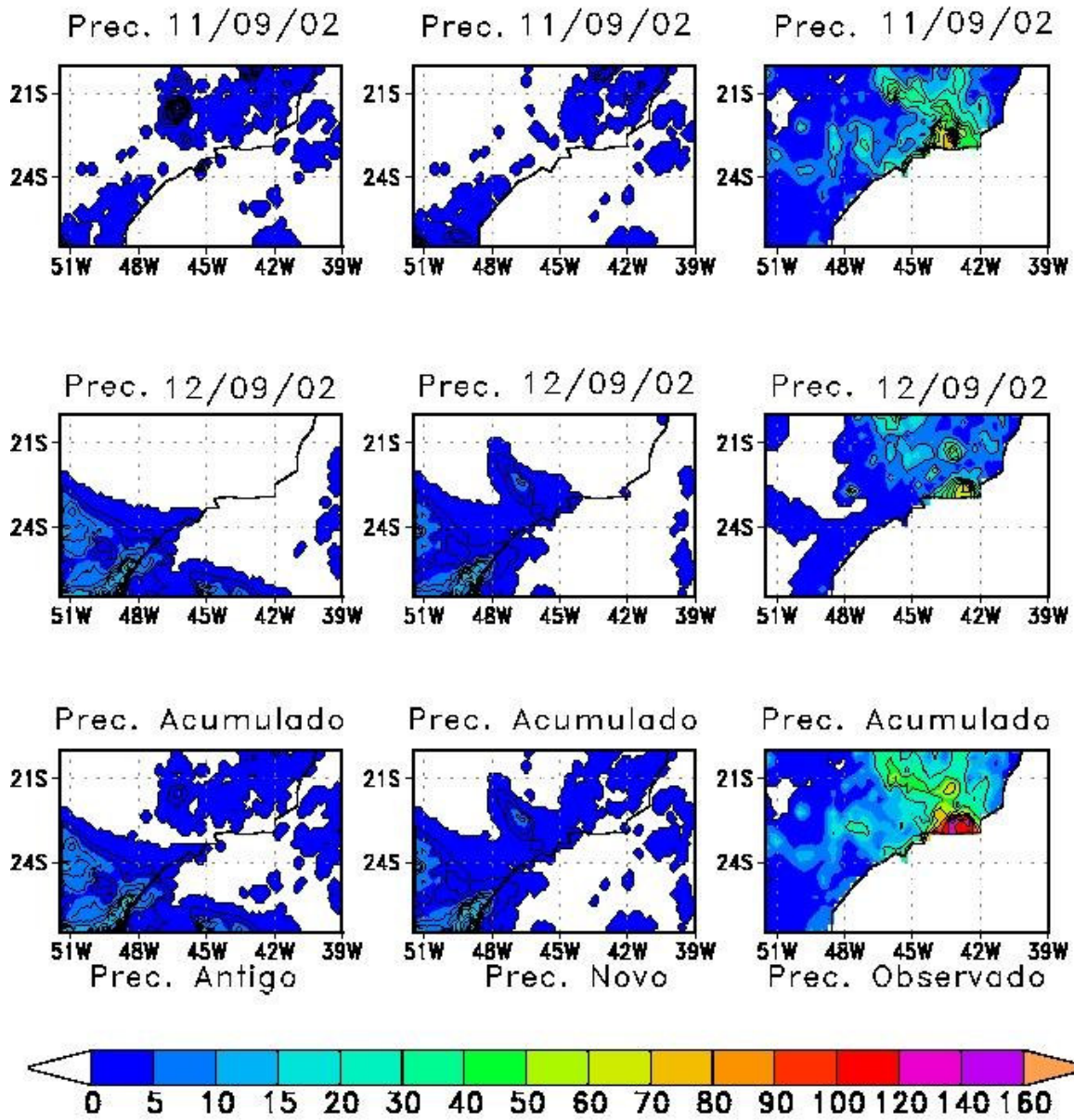
Figura 07 PRECIPITAÇÃO (mm)
