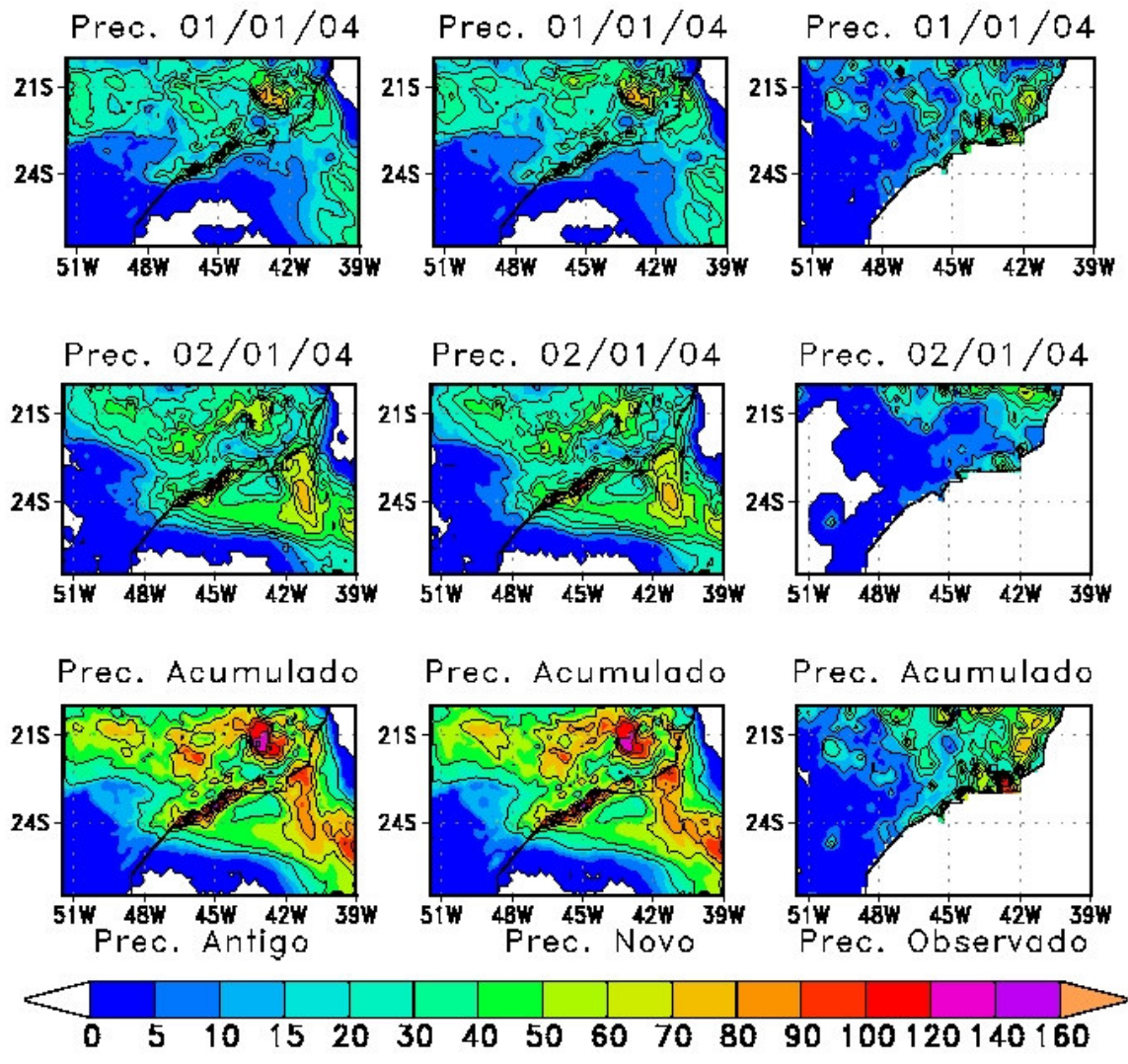
Figura 13 PRECIPITAÇÃO (mm)
