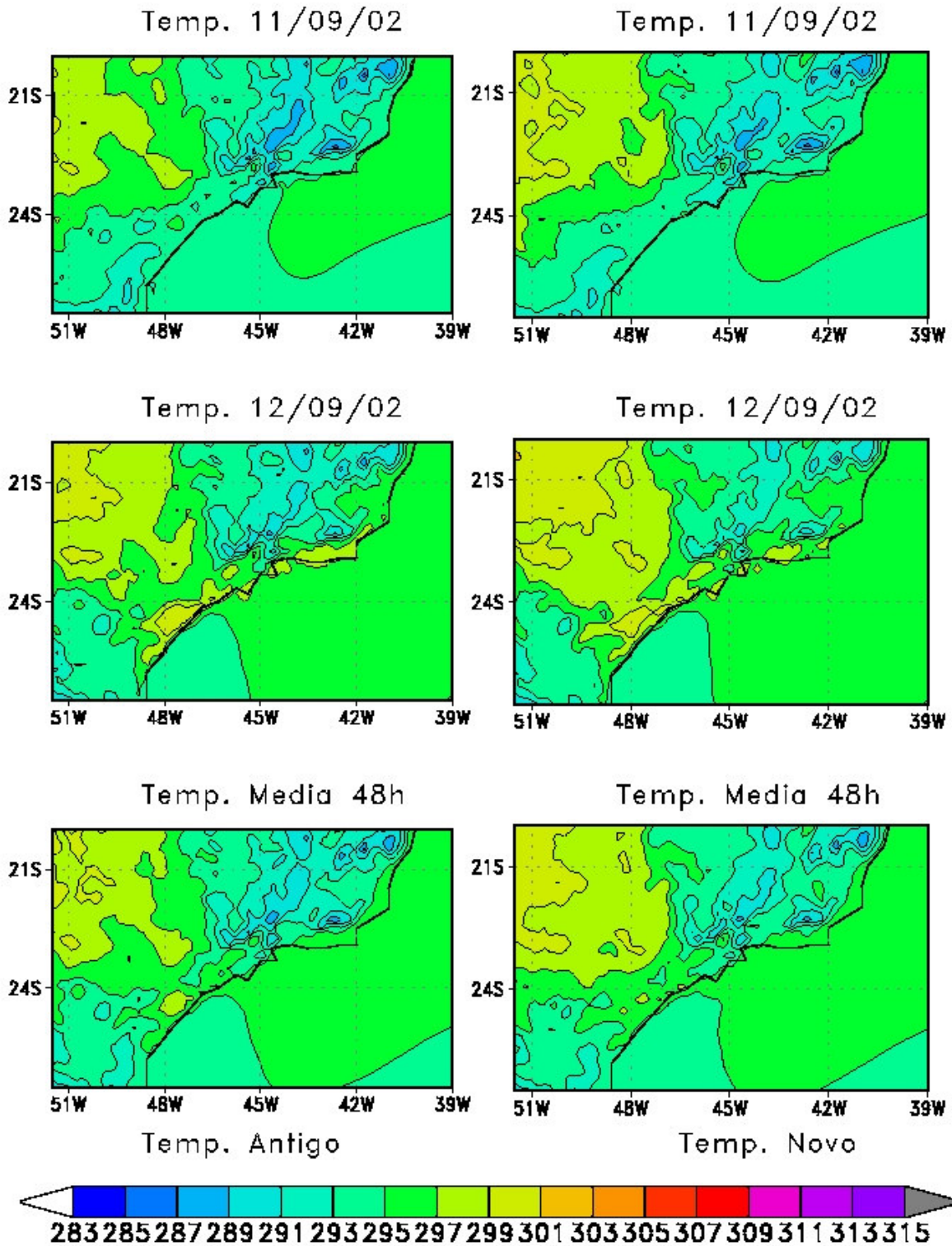
Figura 06 TEMPERATURA (K)
