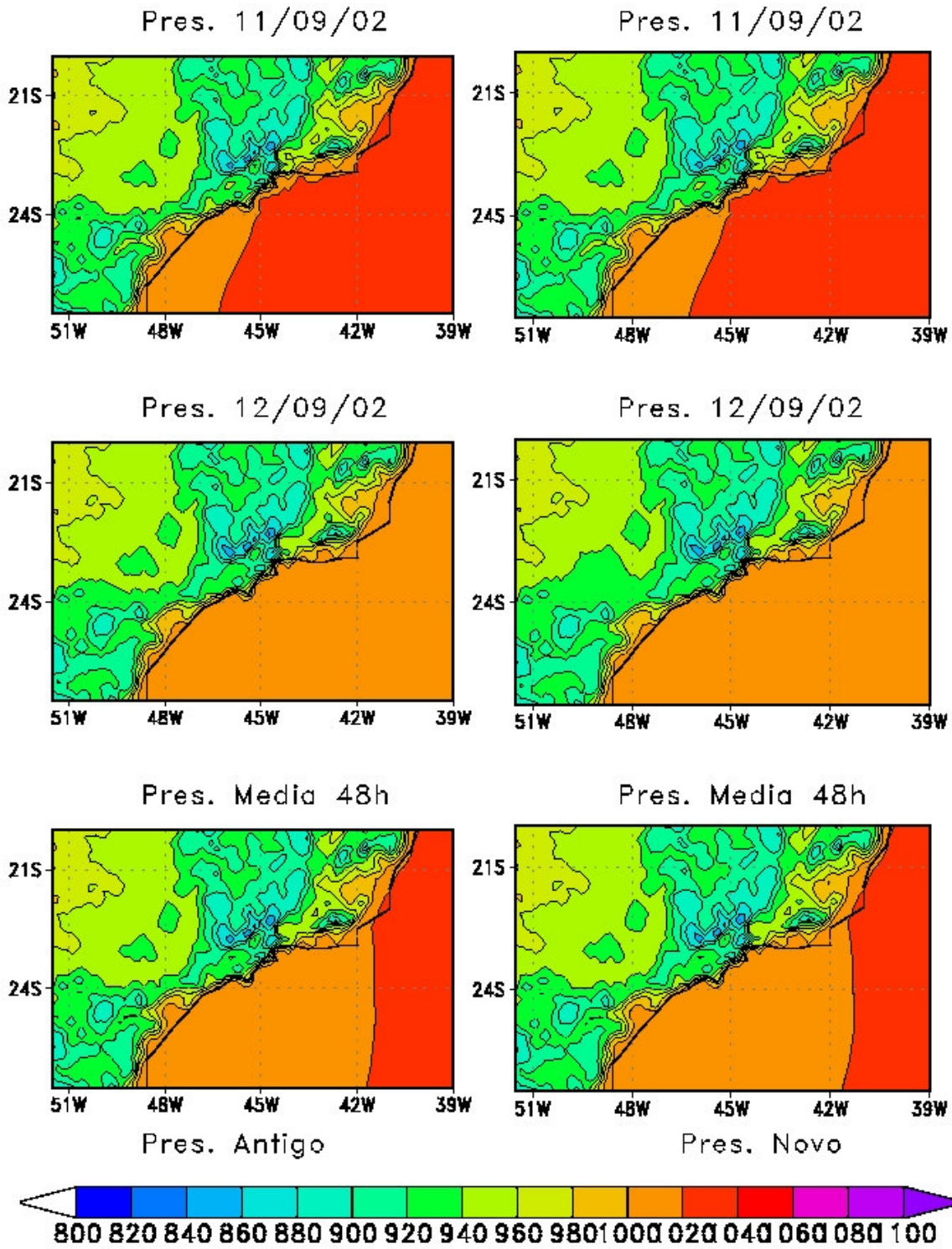
Figura 05: PRESSÃO (Pa)
