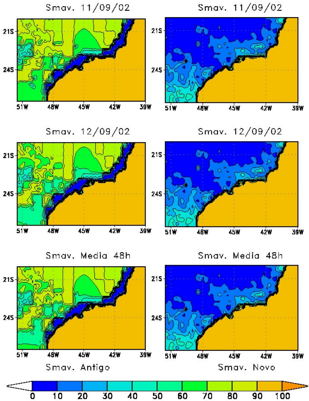
Figura 02: UMIDADE DISPONIVEL DO SOLO(mm)
