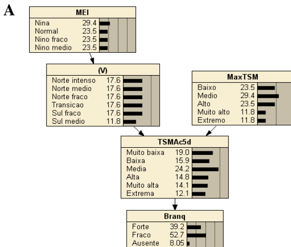
Figura 4.13 - A) Rede Bayesiana 4 e B) tabela de probabilidade condicional do nó branqueamento.
