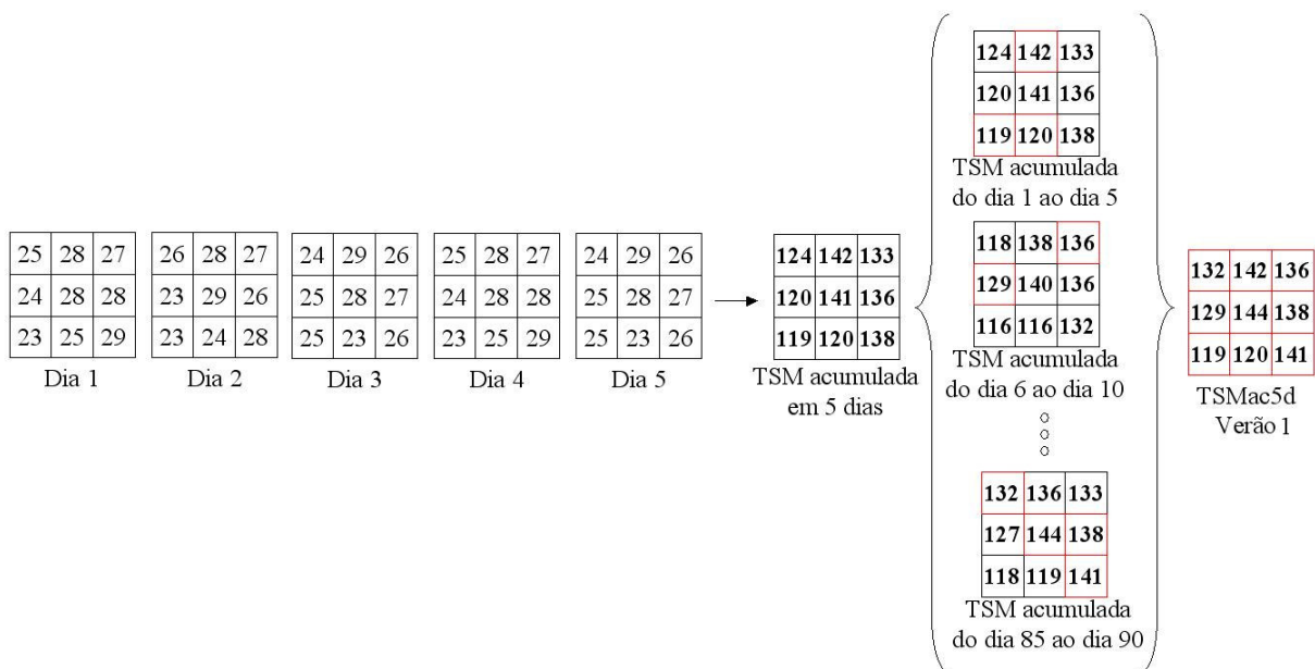
Figura 3.6 - Esquema de construção das imagens de verão da variável Temperatura da Superfície do Mar Acumulada em 5 dias (TSMac5d).
