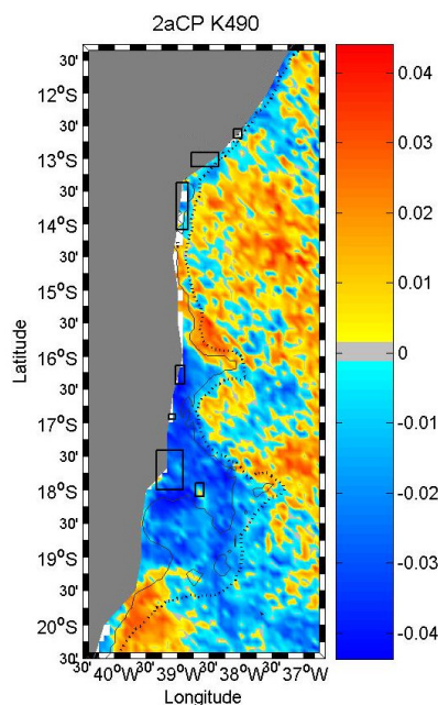
Figura 4.3 - Segunda Componente Principal da série de Coeficiente de atenuação da luz em 490 nm.
