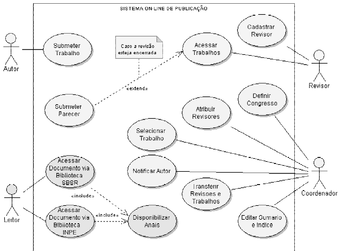
FIGURA 1 – Atores e Serviços envolvidos no Sistema On-line de Publicação.
