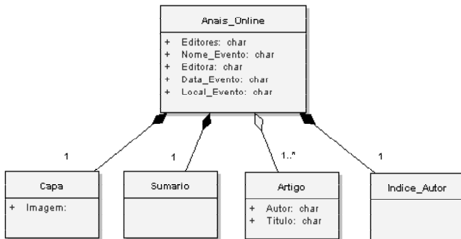
FIGURA 4 – Diagrama de classes representando a estrutura dos Anais.
