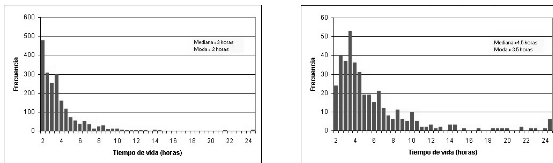
Figura 4: Izquierda: Distribución estadística del tiempo de vida de los SCM para el conjunto total. Derecha: Idem anterior para el conjunto de los sistemas que tuvieron tope fríos durante algún momento de su ciclo de vida.
