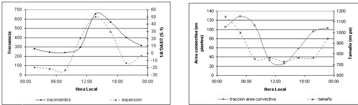
Figura 6: Ciclo diario de las iniciaciones (frecuencia) y la expansión del área (expresado como s^{-1} \cdot 10^6 ) (izquierda) y el tamaño medio de los SCM y su fracción de área convectiva asociada.
