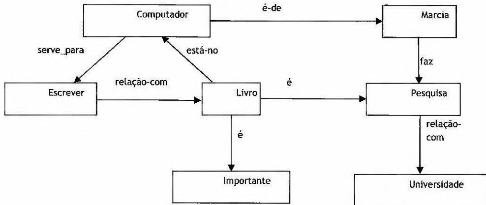
Figura 5.1 – Exemplo de rede semântica.
