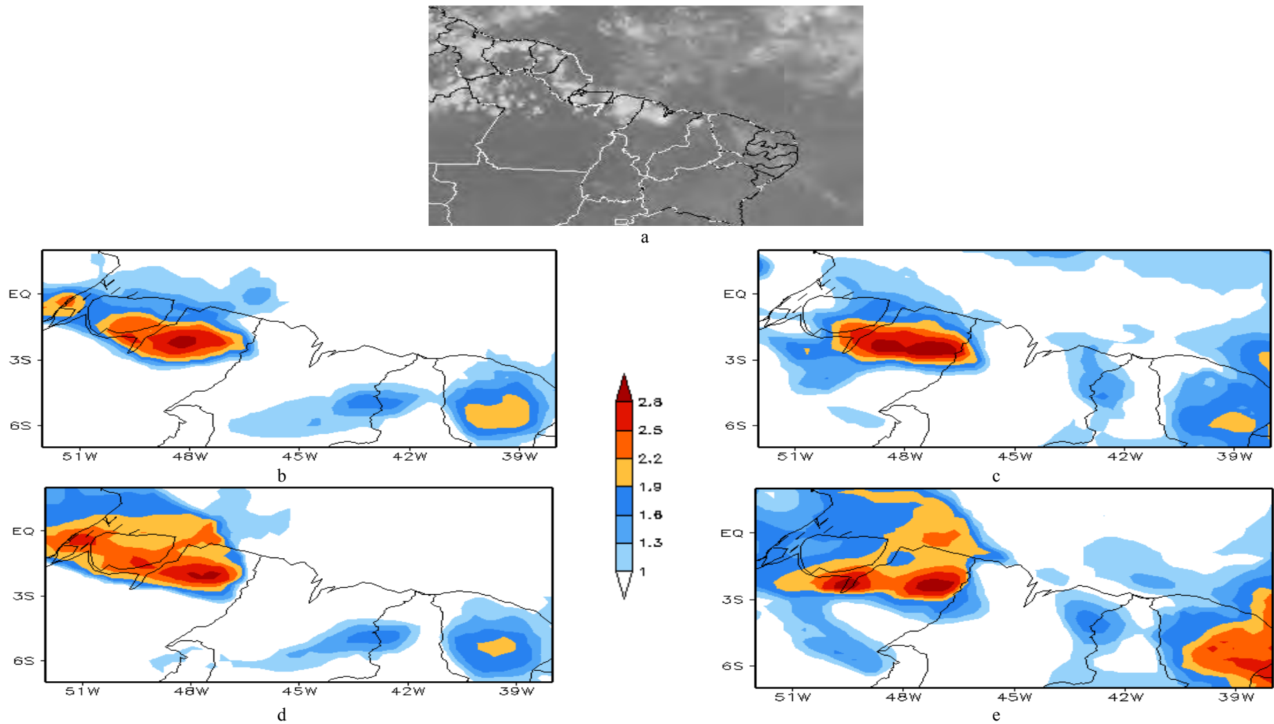
Figura 5.3 – Imagem IR do satélite GOES-12 das 21 UTC do dia 7 de julho de 2005 (a) e campo de FCN simulado das 15 UTC para NCEP1 (b), ERA1 (c), NCEP2 (d) e ERA2 (e).
