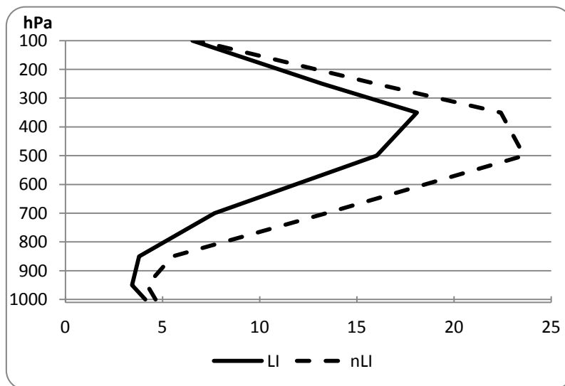
Figura 4.6 – Perfil vertical médio da depressão psicrométrica para as Reanálises.
