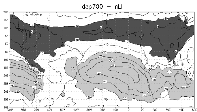
Figura 4.7 – Campos de dep700: média mensal (a), LI (b), nLI (c), diferença entre LI e nLI (d). (Continua)
