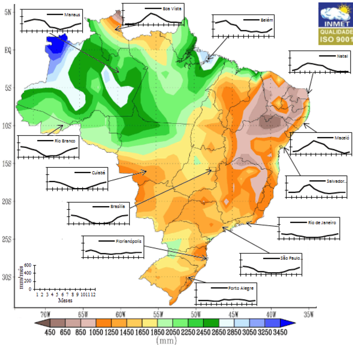
Figura 2.2 – Normais Climatológicas 1961-1990. Precipitação média anual sobre o Brasil e ciclo médio anual sobre algumas Capitais em estudo.
