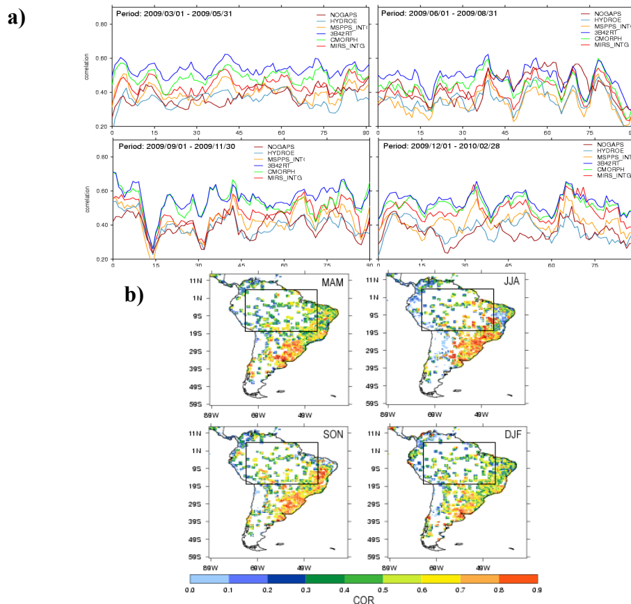
Figura 3.7 – Variabilidade temporal da correlação de diversos produtos de precipitação (a) e distribuição espacial da correlação entre a precipitação observada e a estimada pelo 3B42, para as estações entre o período de março de 2009 à fevereiro de 2010.
