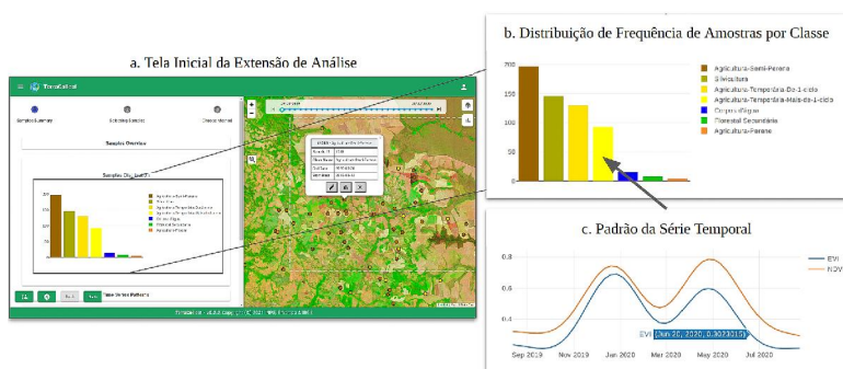
Figura 2. Tela inicial da extensão com a Análise Exploratória de Amostras.
