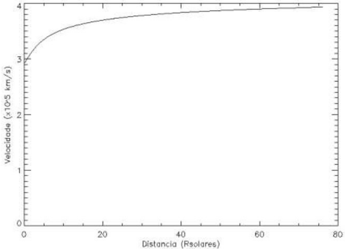
FIGURA 4.18: Perfil central da velocidade da grade de 40x80 R ☉ .
