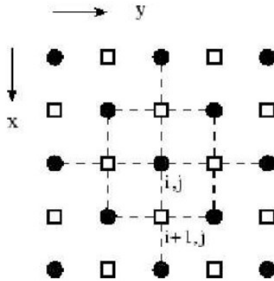
FIGURA 2.3: Primeiro passo em uma malha bidimensional ( \bullet = t_n, t_{n+1} e \square = t_{n+\frac{1}{2}} ).
