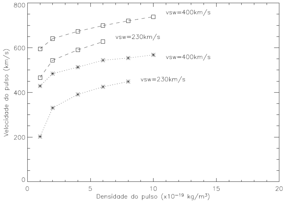
FIGURA 4.14: Velocidade do pulso em função da densidade inicial do pulso para 2 regimes de vento solar (linhas pontilhadas indicam temperatura de pulso de 2 \times 10^6 \text{ K} e linhas tracejadas indicam temperatura de pulso de 6 \times 10^6 \text{ K} ).
