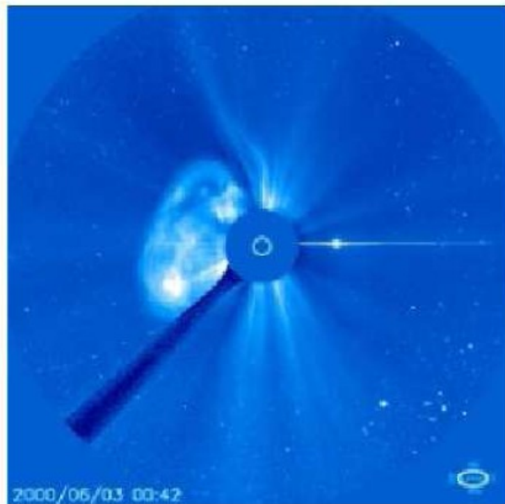
FIGURA 4.11: Comparação da morfologia da EMC simulada com uma EMC observada pelo LASCO.
