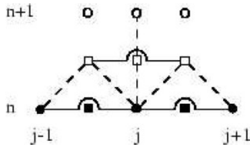
FIGURA 2.4: Segundo passo em uma malha unidimensional.
