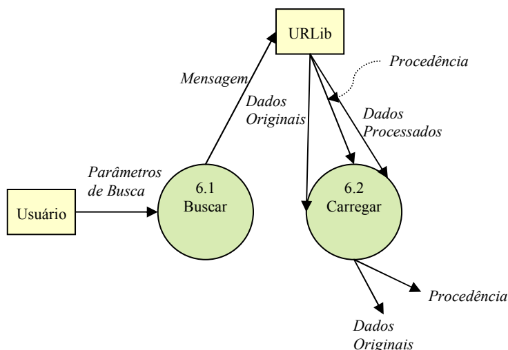
FIGURA 4.11 - Explosão do processo Recuperar.
