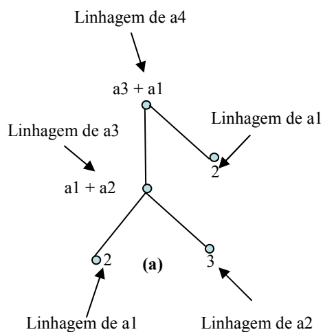
FIGURA 4.6 - Árvore de linhagem para obtenção de a4 .
