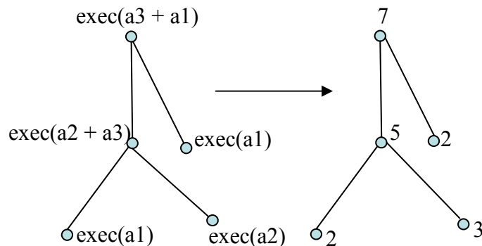
FIGURA 4.14 - Execução dos nodos da árvore de linhagem para obtenção dos dados.
