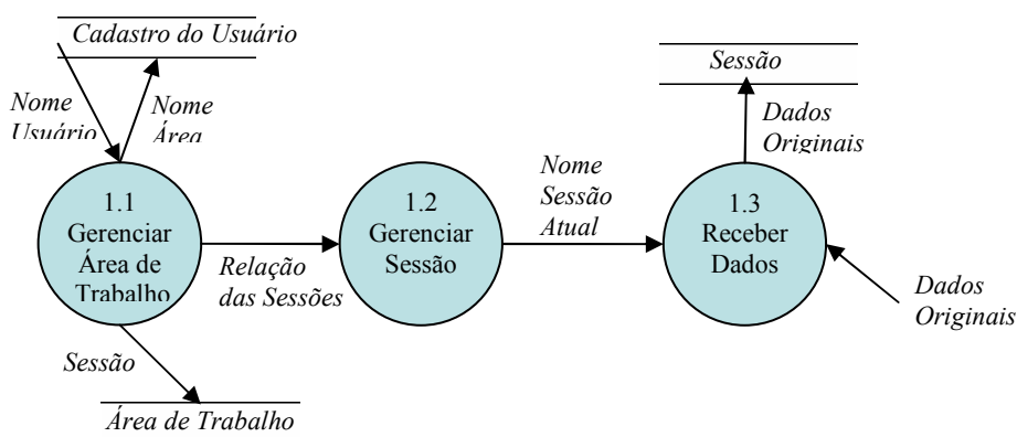
FIGURA 4.3 – Explosão do processo Acessar.
