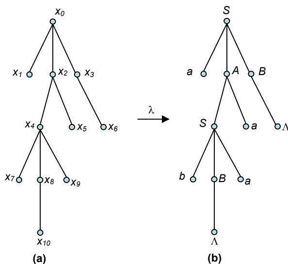
FIGURA 2.1- (a) e (b) Árvores representando uma gramática de livre-contexto. FONTE: adaptado de (Harrison, 1978).
