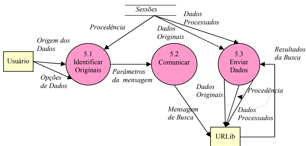
FIGURA 4.8 - Explosão do processo Armazenar.
