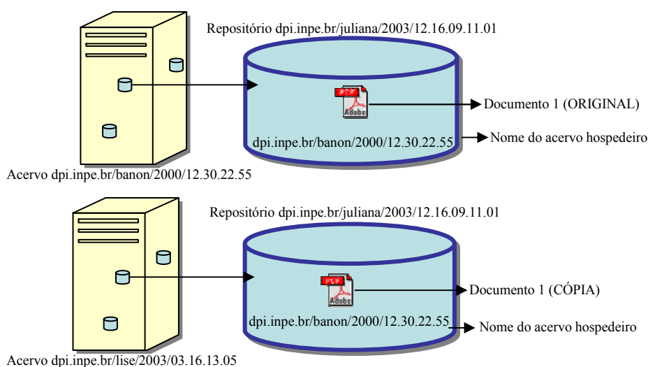
FIGURA 3.9 - Identificação dos documentos originais pela URLib .
