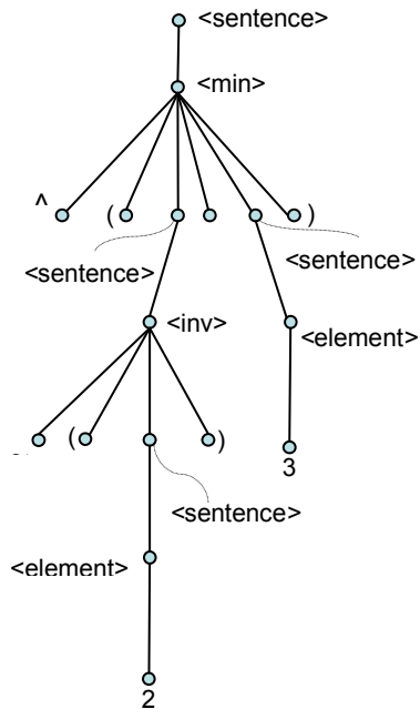
FIGURA 2.4 - Árvore de derivação para a geração da frase \wedge(\sim(2) 3) .
