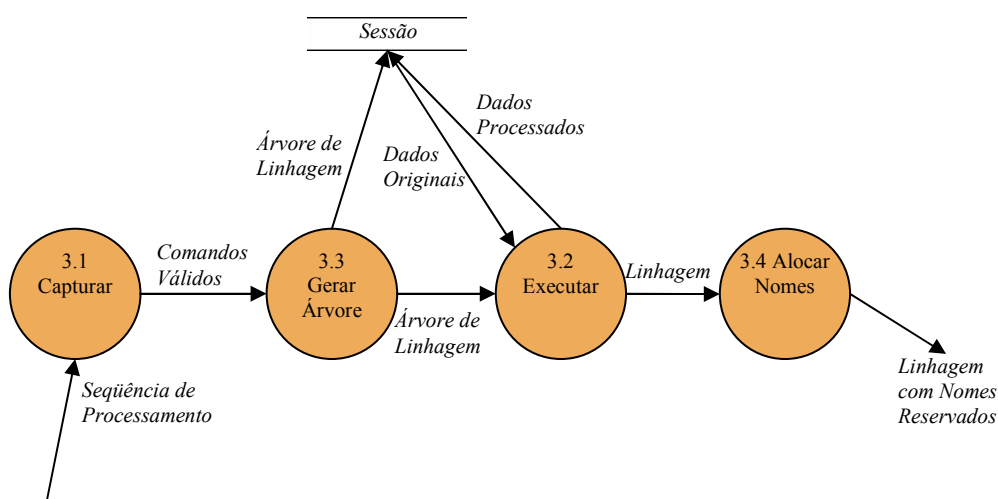
FIGURA 4.5 – Explosão do processo Processar.
