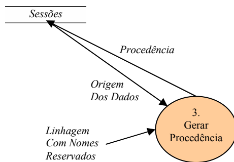
FIGURA 4.7 - Processo Gerar Procedência.
