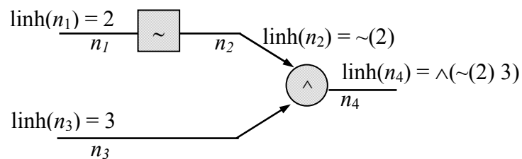
FIGURA 2.10 - Alocação de nomes reservados às linhagens.
