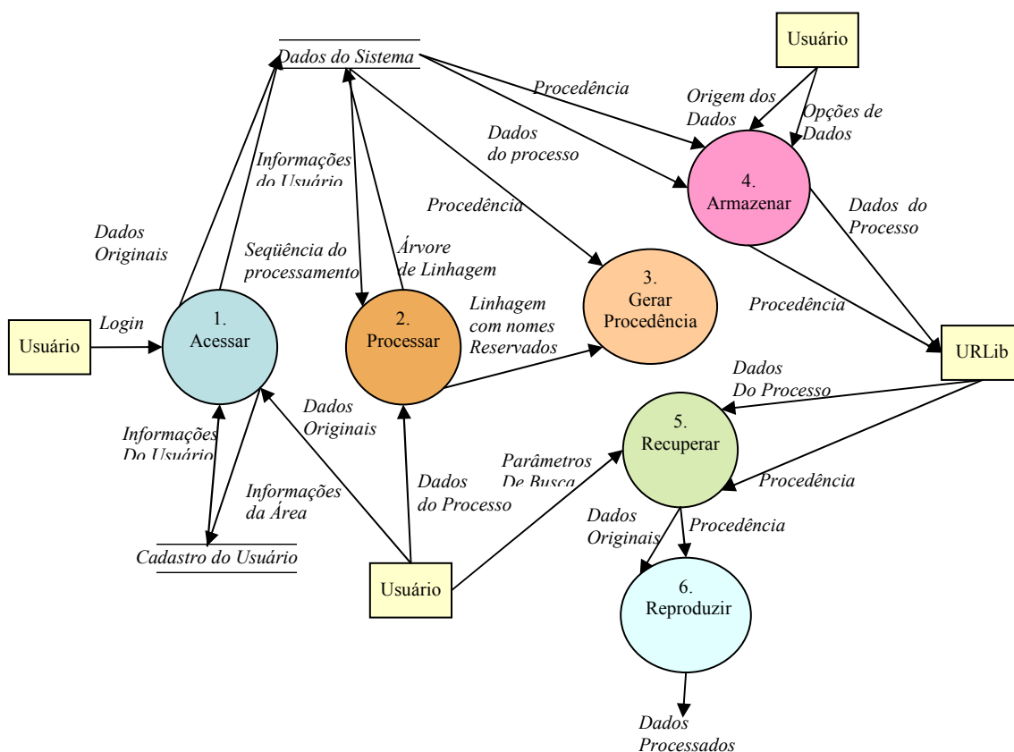
FIGURA 4.2 – Diagrama de fluxo de dados do SGPD.
