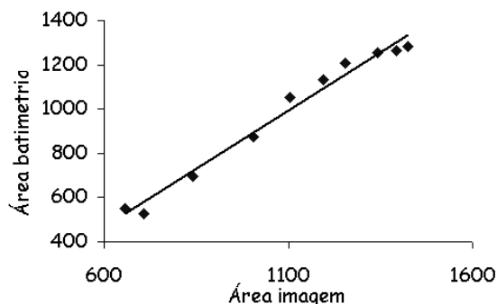
Fig. 13 - Correlação entre áreas inundadas obtidas a partir de imagens TM/Landsat e a partir de dados batimétricos (Fonte: BARBOSA, 2005)
