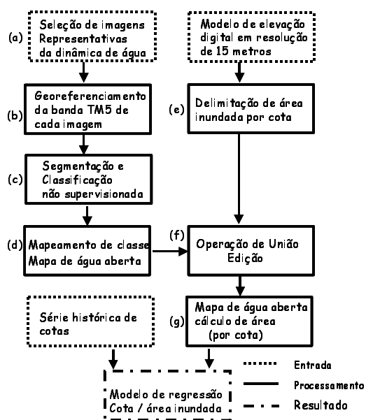
Fig. 9– Seqüência de processamento para modelagem da dinâmica de área inundada (Fonte: BARBOSA, 2005).
