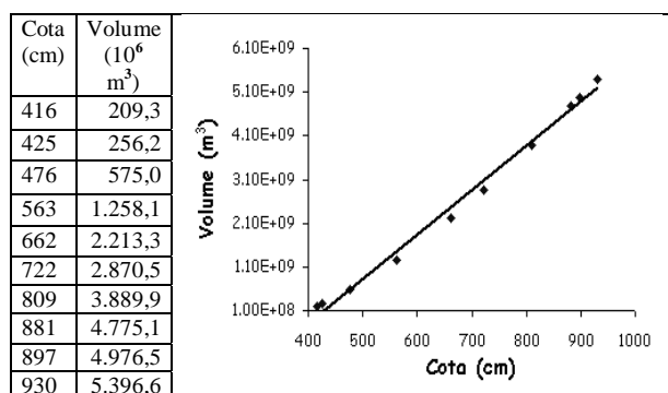
Fig. 17 – Volume de água na planície para diferentes cota e modelo relacionando cota com volume (Fonte: Barbosa, 2005)
