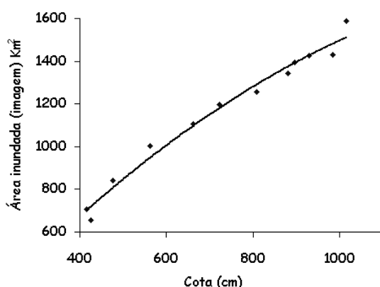
Fig. 11 - Modelo de regressão relacionando cota com área de água aberta, obtida a partir imagens.
