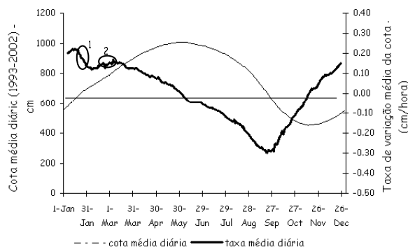
Fig. 10 – Taxa de variação do nível da água. (Fonte: BARBOSA, 2005)
