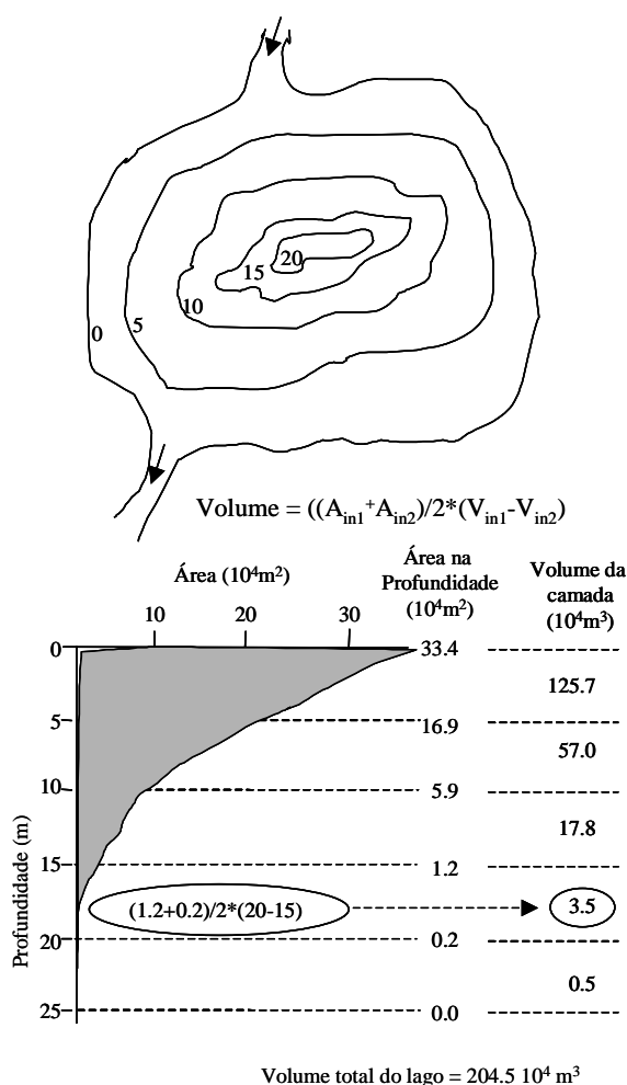
Fig. 14– Método para determinação do volume de um lago (Adaptado de KALFF (2001))
