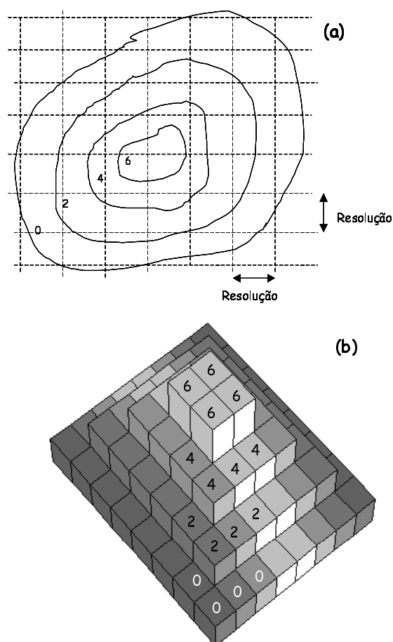
Fig. 15 – Método para determinação do volume de um lago através de uma grade regular de células. (a) – A região de interesse é particionada em células regulares. (b) – Representação 3D onde cada célula recebe o valor médio de profundidade.
