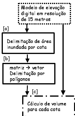
Figura 16 – Sequência de processamento para a dinâmica de volume. (Fonte: BARBOSA, 2005)
