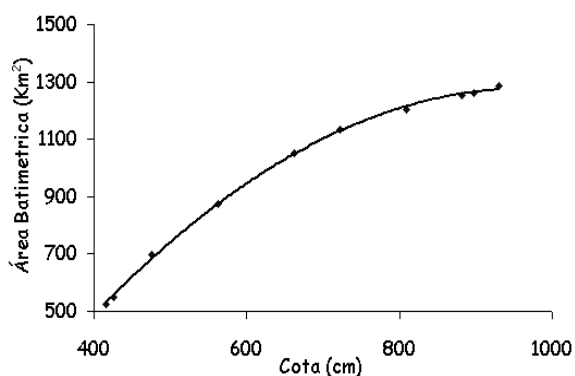
Fig. 12 - Modelo de regressão relacionando cota com área de água aberta, obtida a partir de dados batimétricos.
