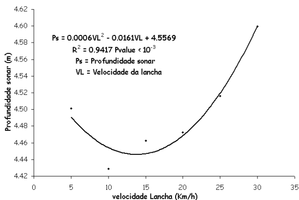
Fig. 6 – Modelo de correção da profundidade em função da velocidade da lancha (Fonte: BARBOSA, 2005)
